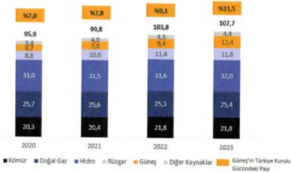
Grafik: Kaynaklara Göre Türkiye Elektrik Kurulu Gücü (GW)
