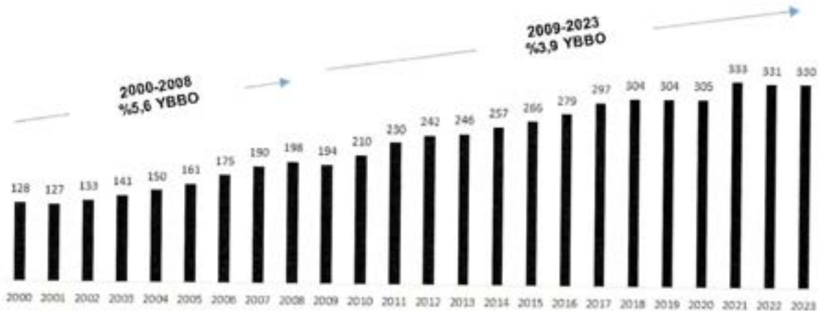
Grafik: Brüt Elektrik Talebi (TWh, 2000-2023)
