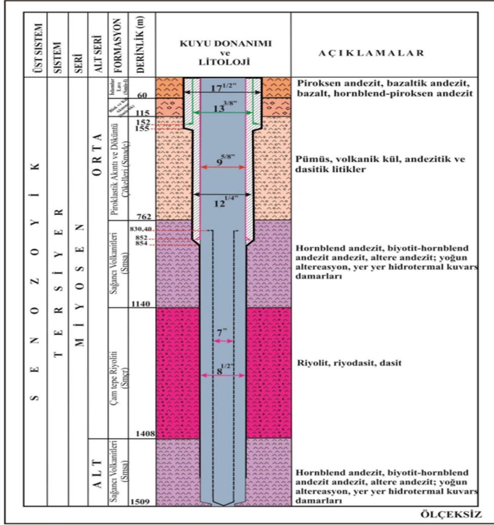
Şekil 19: SA1-Kuyu Logu Ve Teçhizi
