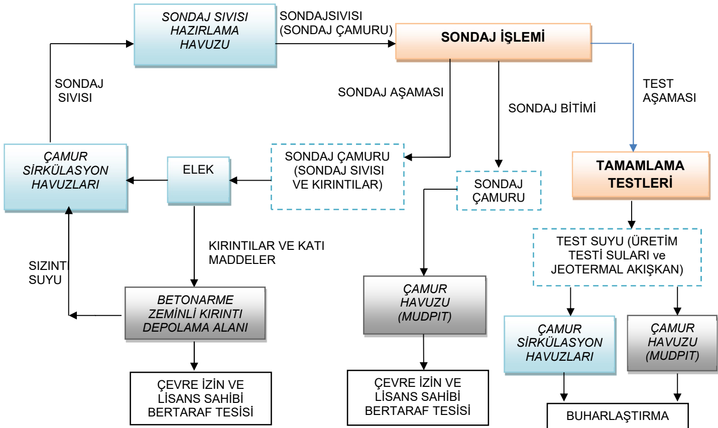
Şekil 48: Sondaj İşlemi Sıvı Atık Akış Diyagramı
